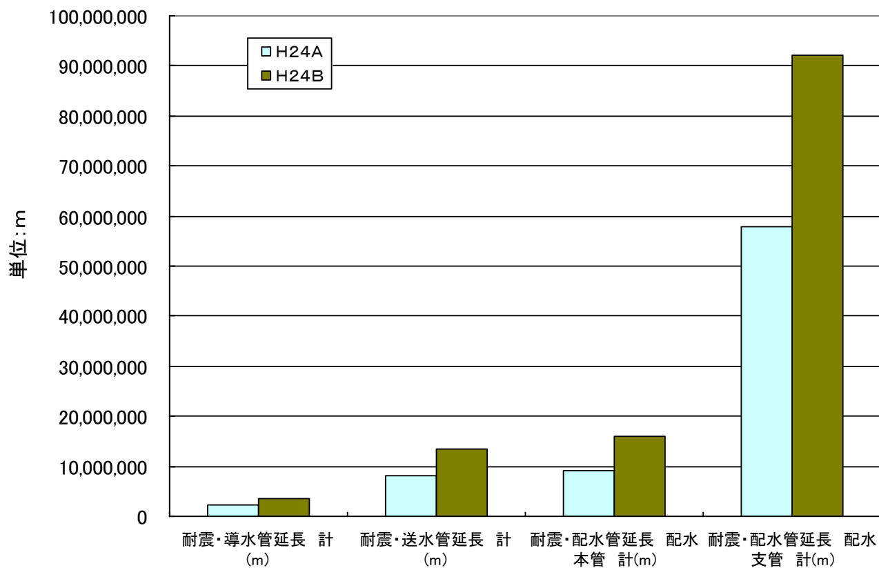
図3-2 耐震管・管路延長の推移(全国、上水+用供)
