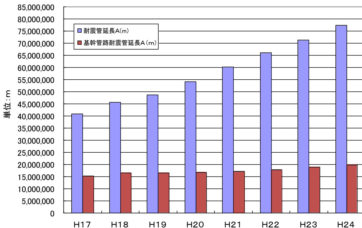
図1-1 耐震管延長A及び基幹管路耐震管延長Aの推移 (全国、上水+用供)
