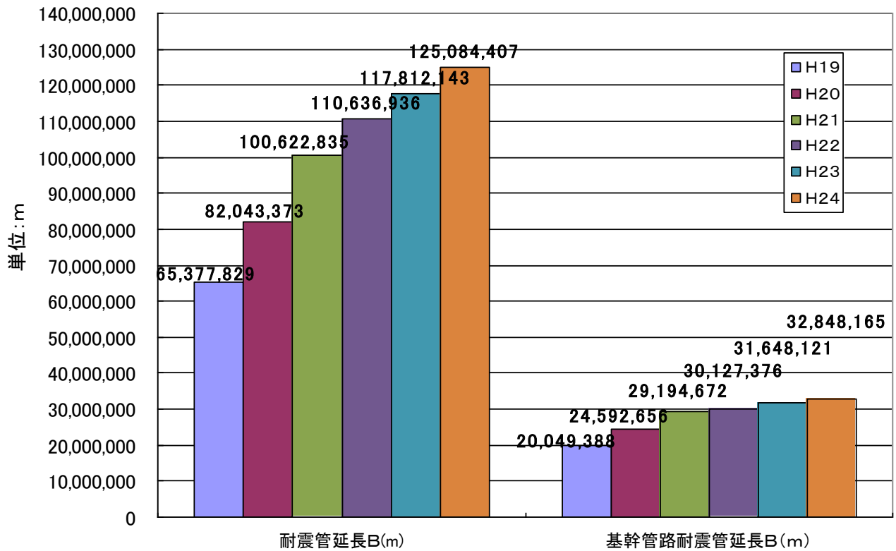
図2-1 耐震管延長B及び基幹管路耐震管延長Bの推移 (全国、上水+用供)
