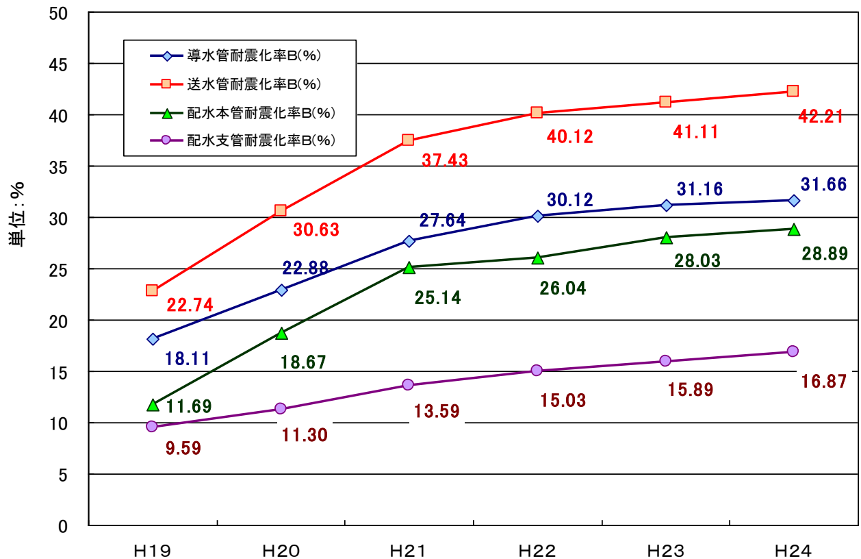
図2-4 導水管・送水管・配水本管・配水支管別にみた耐震化率Bの推移 (全国、上水+用供)
