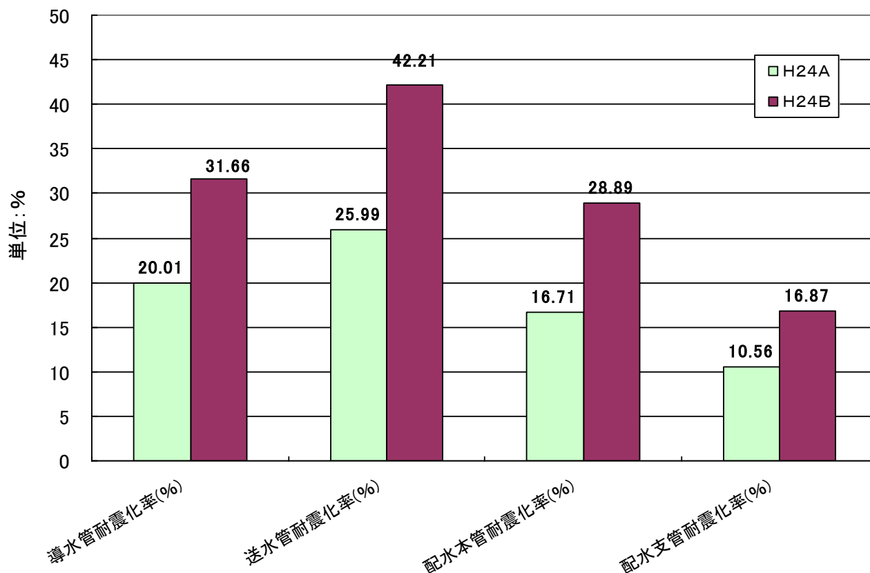
図3-4 導水管・送水管・配水本管・配水支管別にみた管路耐震化率 (全国、上水+用供)
