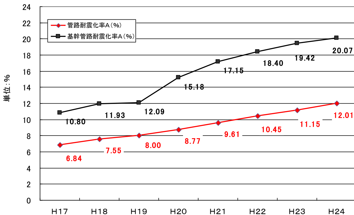
図1-2 管路耐震化率A及び基幹管路耐震化率Aの推移 (全国、上水+用供)
