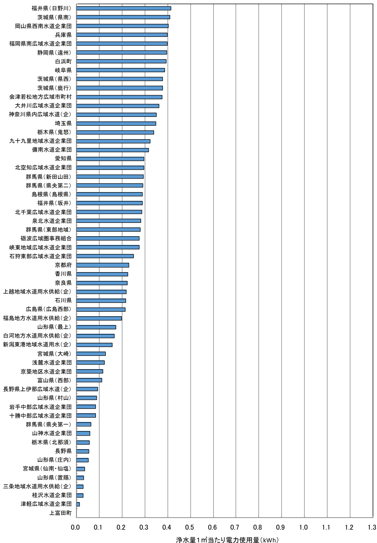
図4-1-2 浄水量1m 3 当たり電力使用量 (平成24年度、水道用水供給事業)ーその2ー
