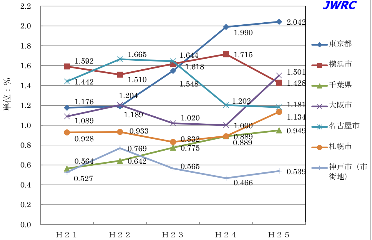
(参考図 1) 規模の大きい上水道事業者における管路更新率の推移 (その 1)
