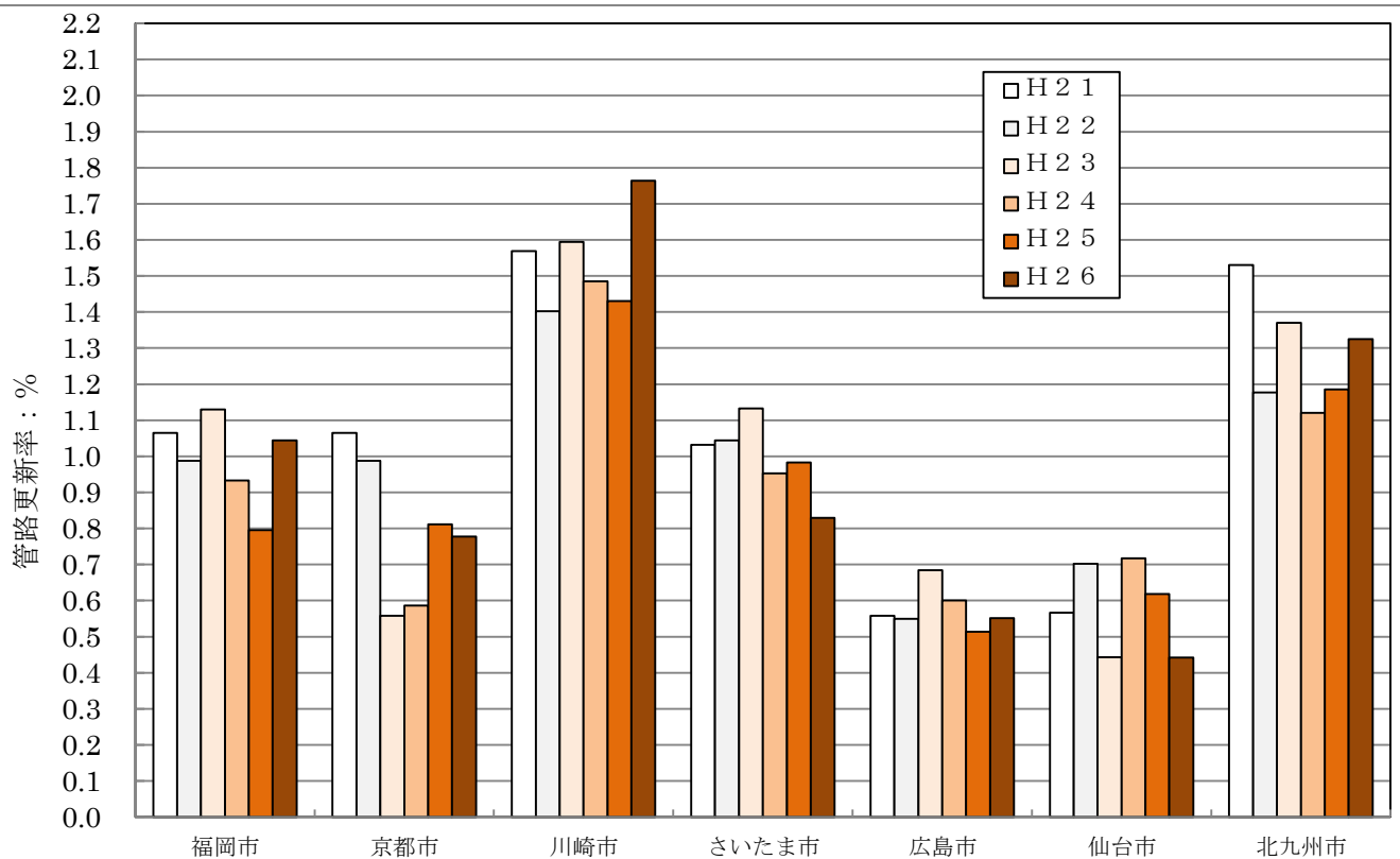
(参考図2) 規模の大きい上水道事業者における管路更新率の推移 (その2)
