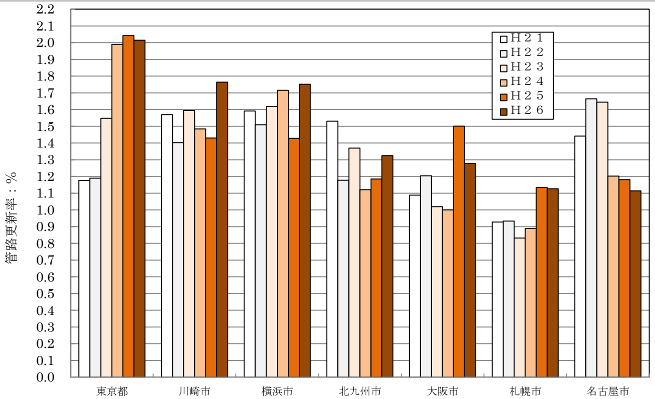
(参考図1) 規模の大きい上水道事業者における管路更新率の推移 (その1) -平成26年度の管路更新率が高い順-
