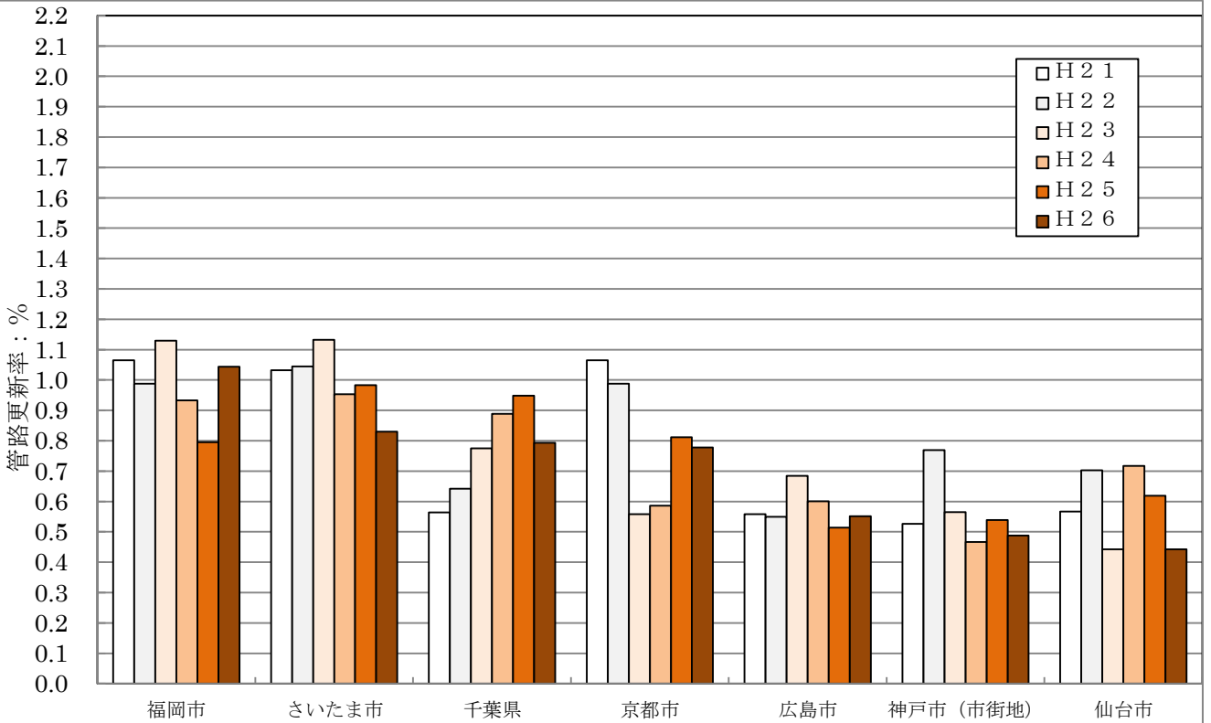
(参考図2) 規模の大きい上水道事業者における管路更新率の推移 (その2) -平成26年度の管路更新率が高い順-
