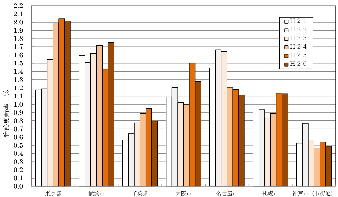
(参考図1) 規模の大きい上水道事業者における管路更新率の推移 (その1)
