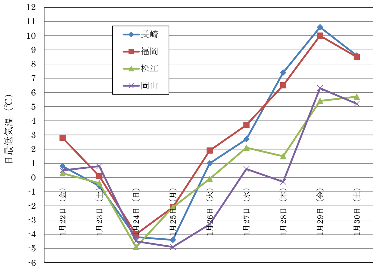
図1 日最低気温の推移 (平成28年1月、気象庁データ)
