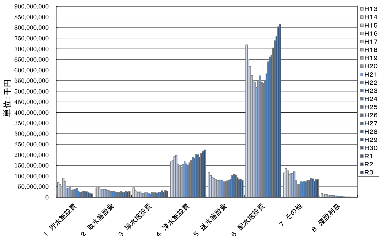
図1－3 施設別事業費(全国、上水＋用供、施設別)
