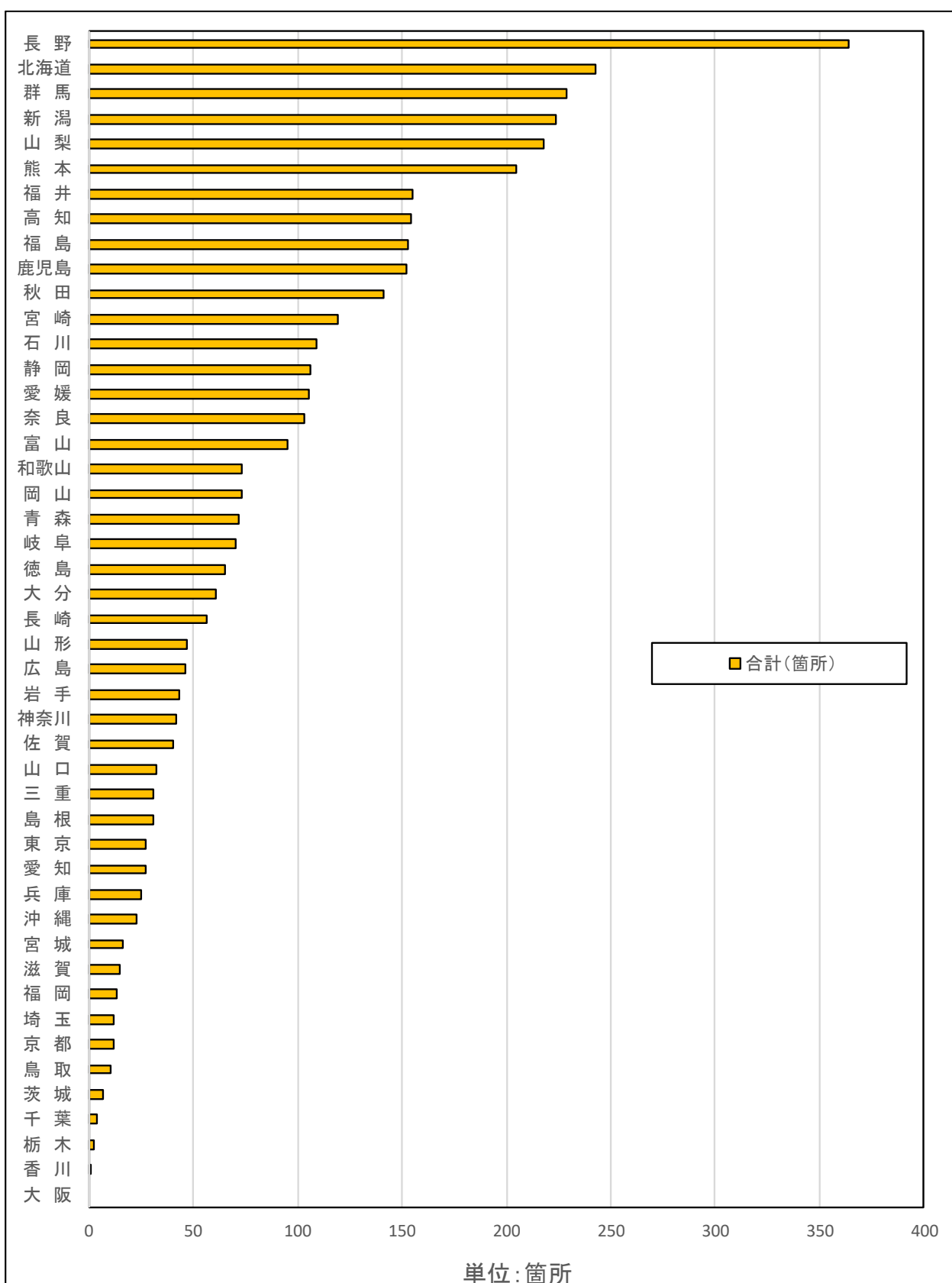
図3-1 簡易水道事業における浄水施設数 —合計(箇所)、令和3年度—
