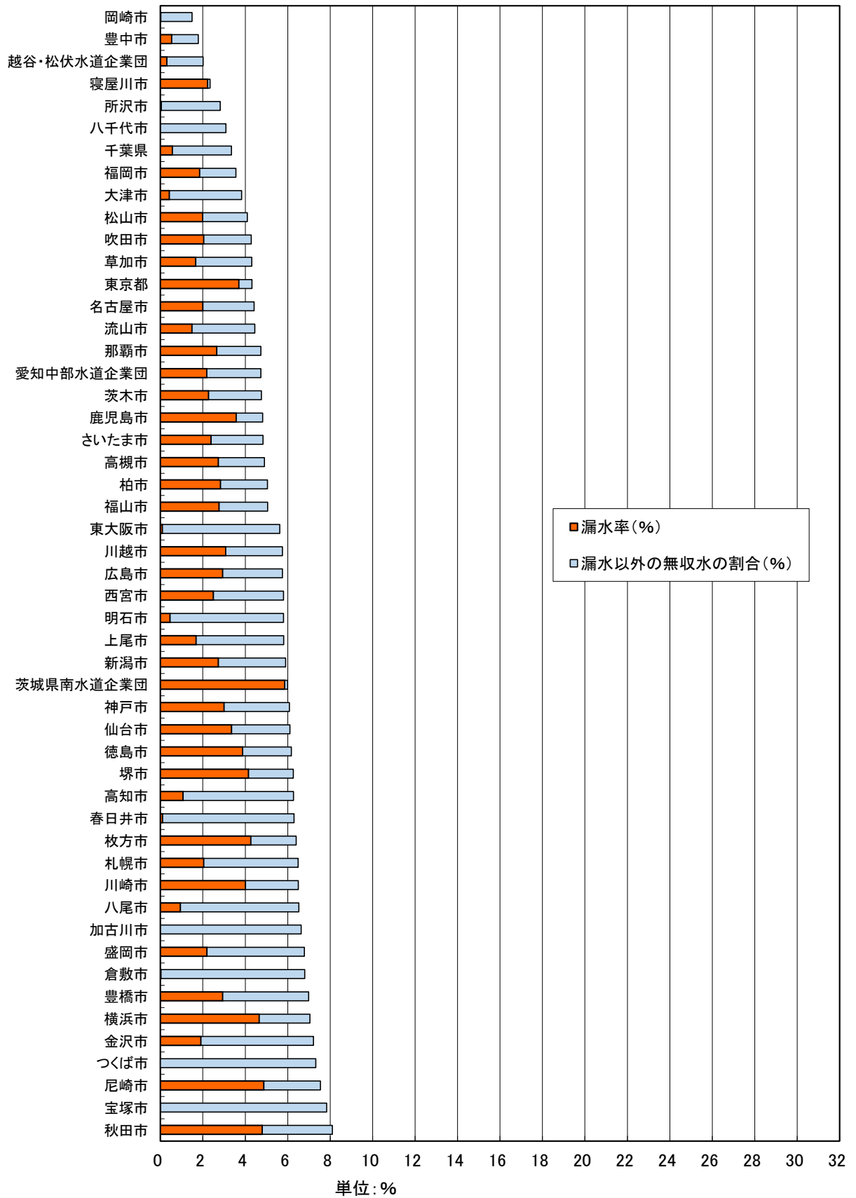
図2-1 現在給水人口20万人以上の上水道102事業者の無収水率 (令和4年度、無収水率の低い順)
