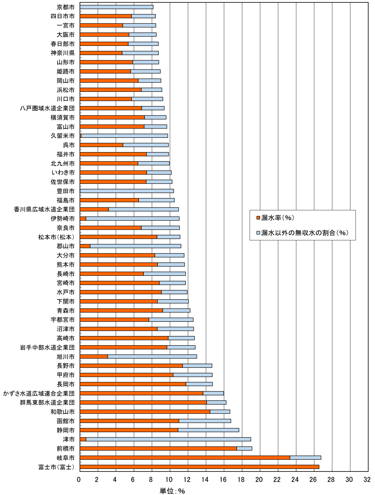
図2-2 現在給水人口20万人以上の上水道102事業者の無収水率 (令和4年度、無収水率の低い順)
