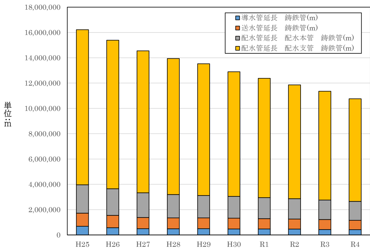
図1-1 鋳鉄管の残存延長の推移(全国、用供+上水、積上げ)
