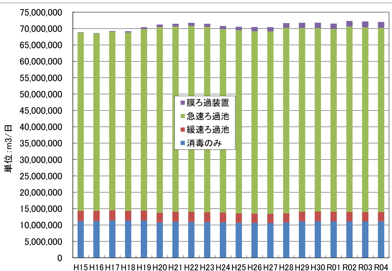
図2-1 浄水方法別計画浄水量の推移(用供+上水)ー積み上げー JWRC
