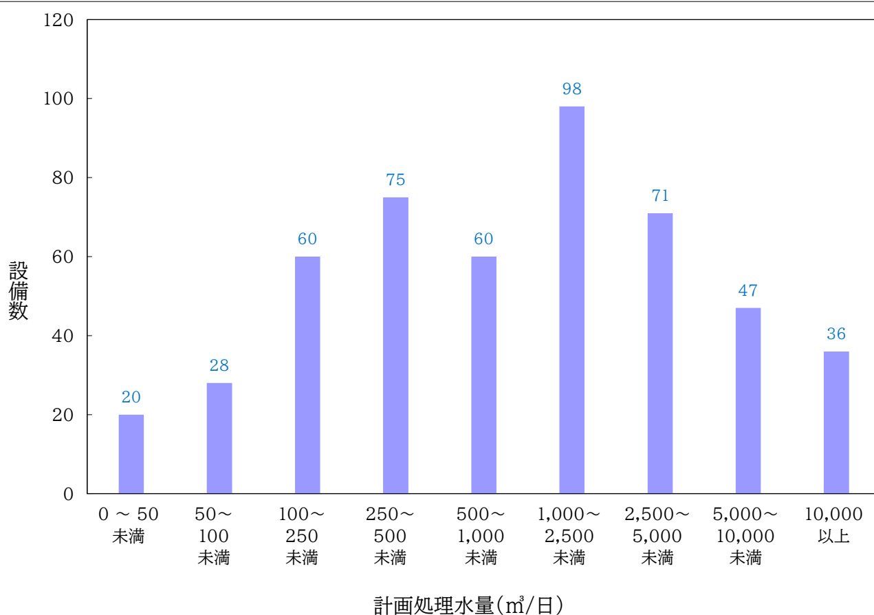
図2 浄水プロセスにおける紫外線処理設備の計画処理水量別設備数
