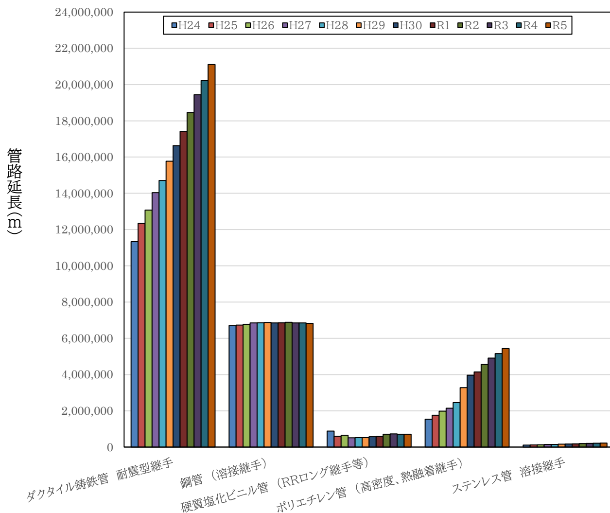
図3 基幹管路における管種別耐震管延長の年度別推移
